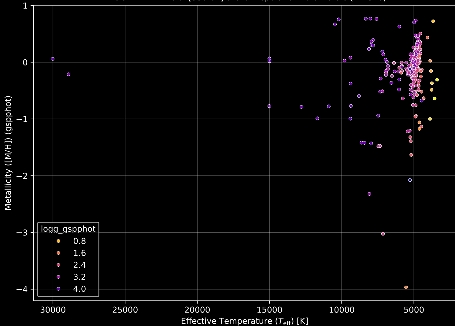
APOGEE DR17 Field: [350-04] Stellar Population Parameters (n= 328)
